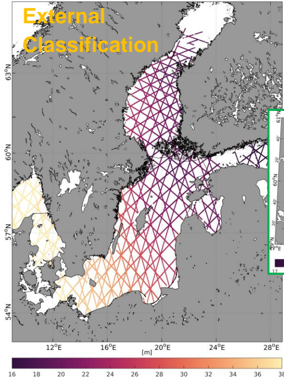
Example: Sea Surface Heights ALES+ 2009-04 (Jason1-EM, Jason-2, Envisat)
