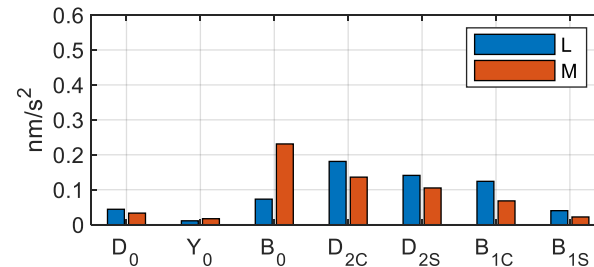
ECOM2
