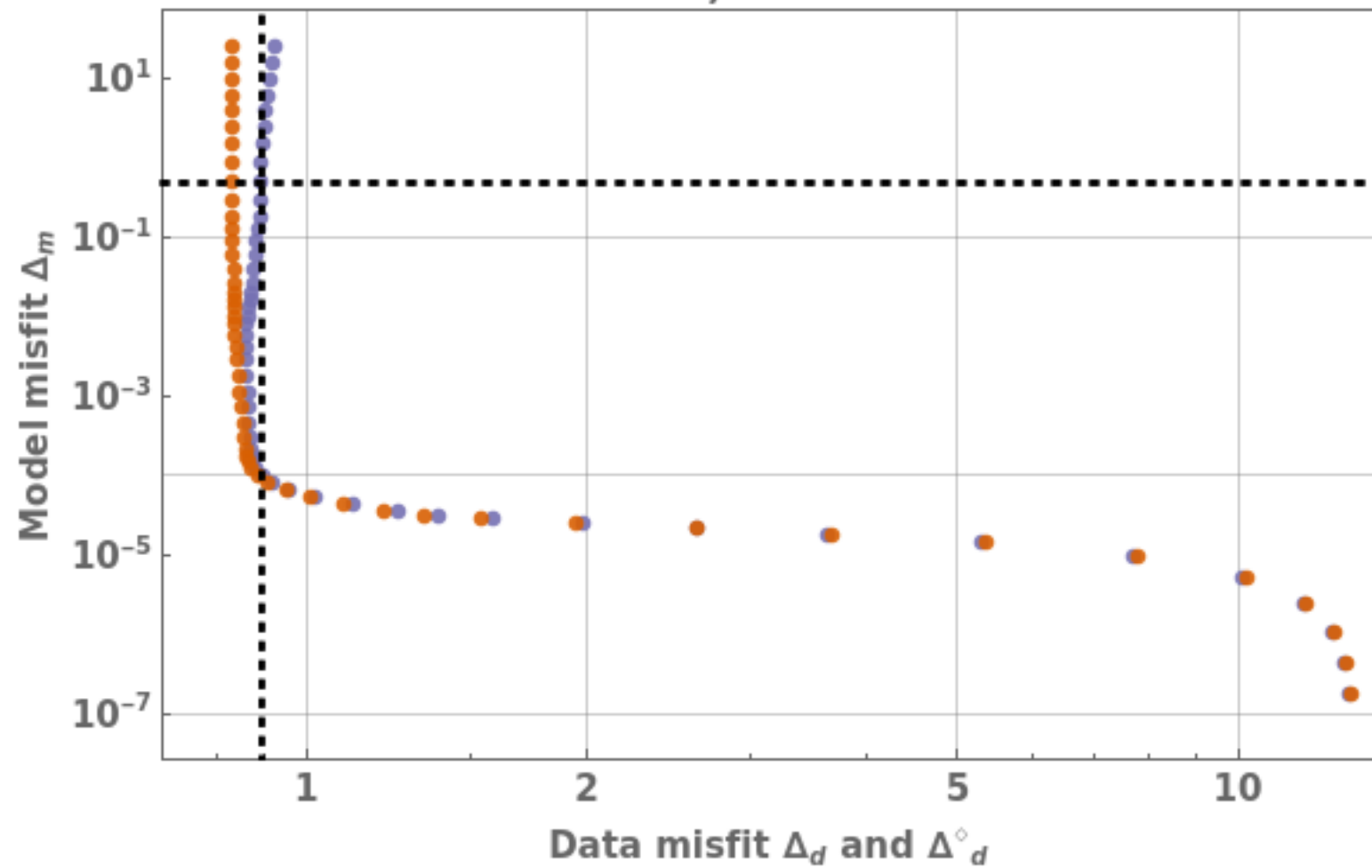
Misfit curve, \alpha: 0.000398107
