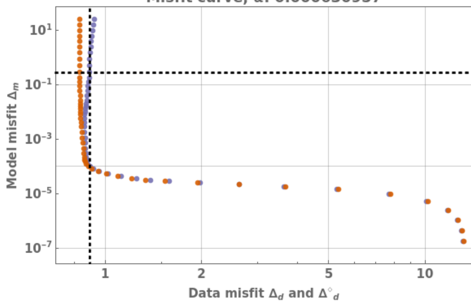
Misfit curve, \alpha : 0.000630957
